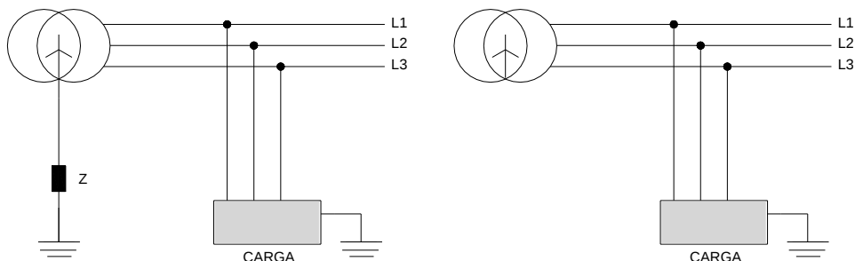
Figura 5 - Esquema IT
