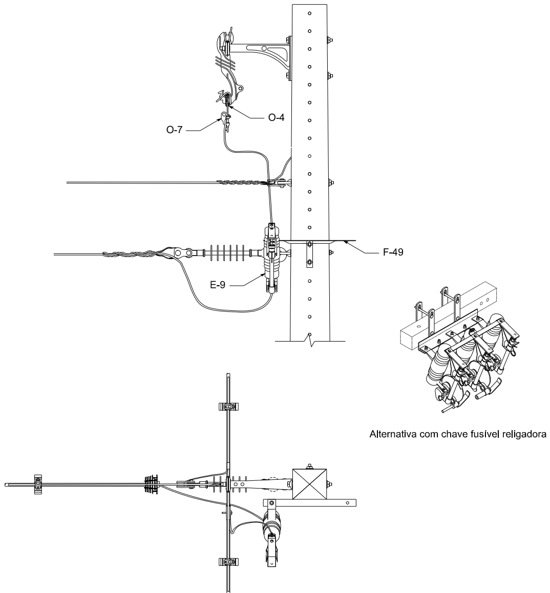
Figura 48 – Instalação de equipamento – Chave fusível em derivação monofásica - Estrutura monofásica
