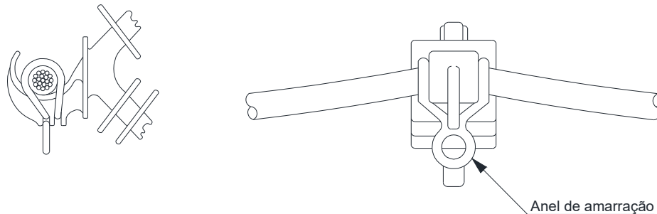
Figura 89 – Amarrações e ligações – Amarração do cabo protegido em espaçador monofásico, vertical e losangular – Anel de Amarração
